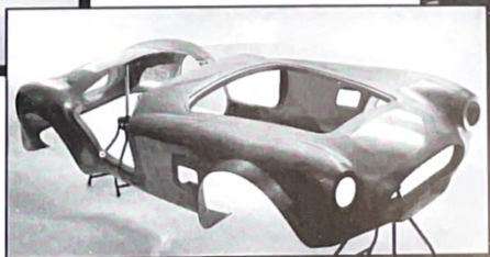
HI-TECH 289FIA ALUMINUM BODY SHELL
